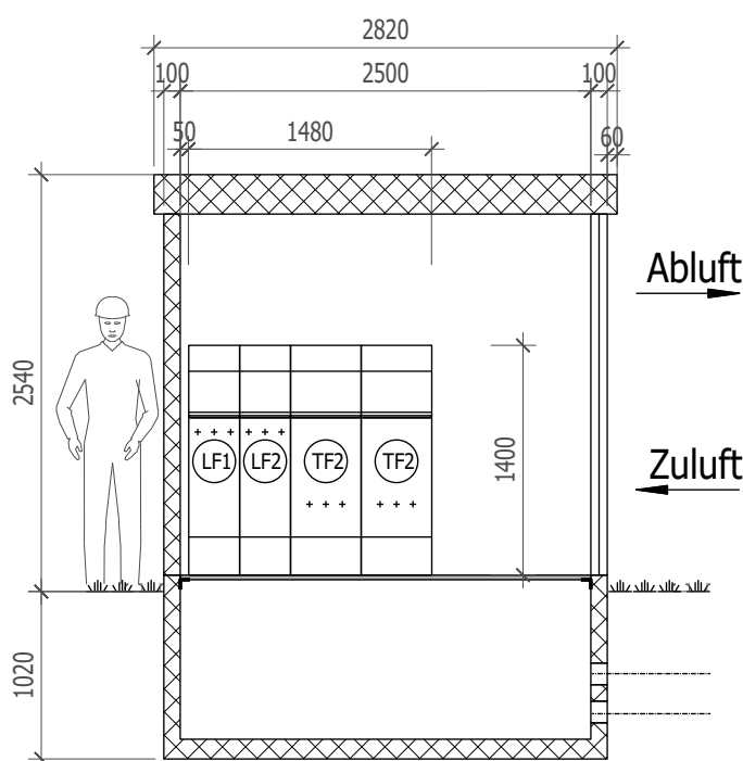
Schnitt C-C
