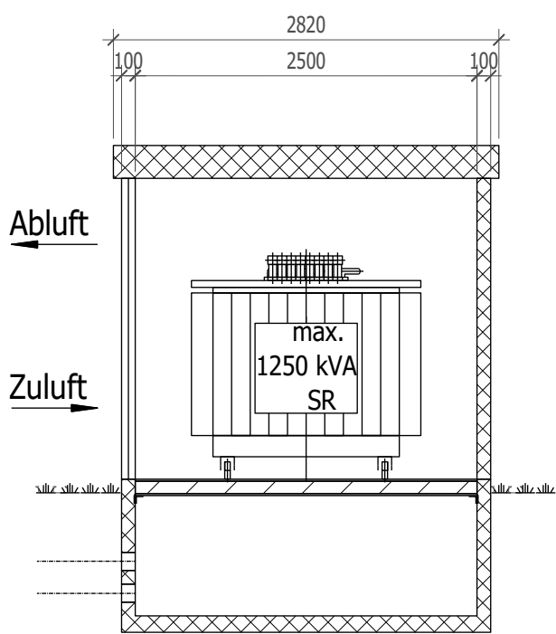
Schnitt A-A
