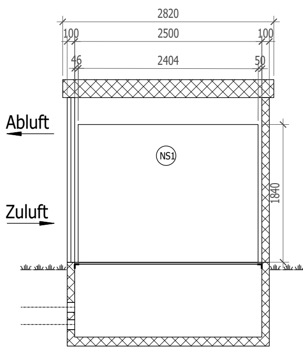
Schnitt B-B
