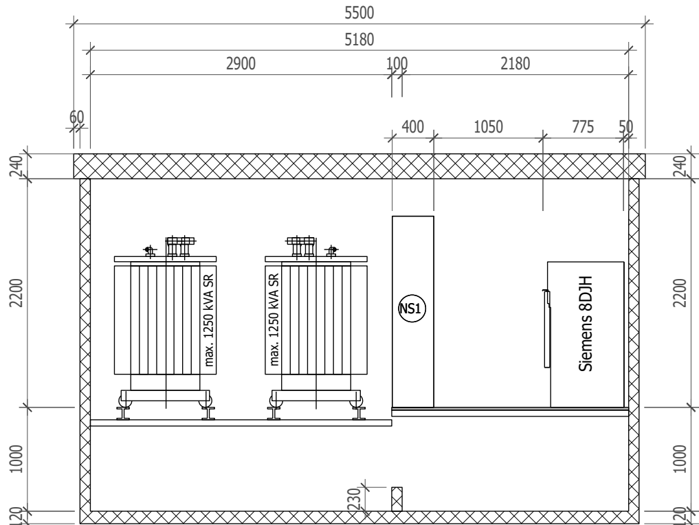
Schnitt D-D
