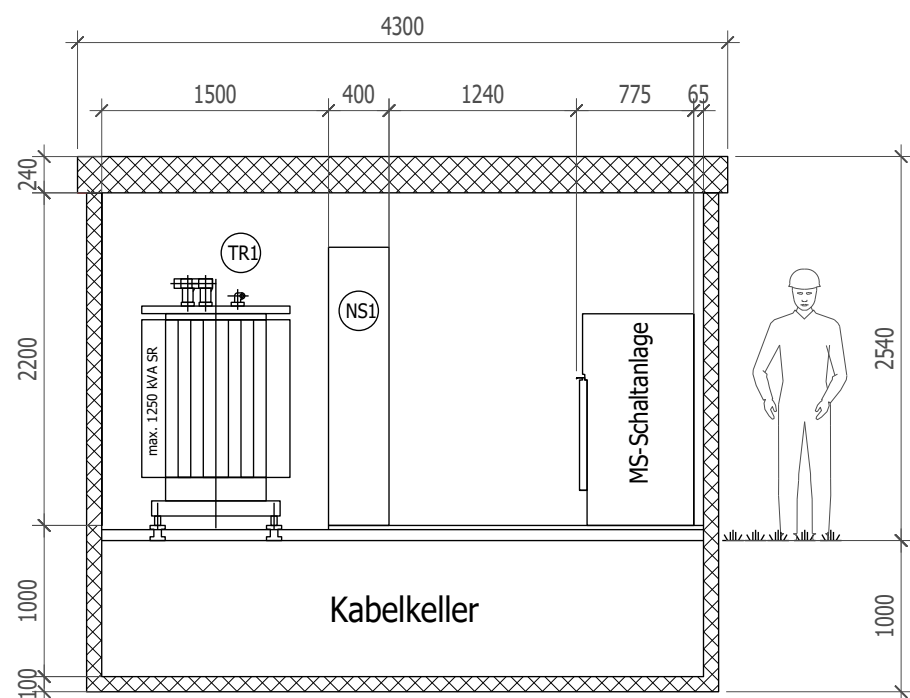
Schnitt B-B
