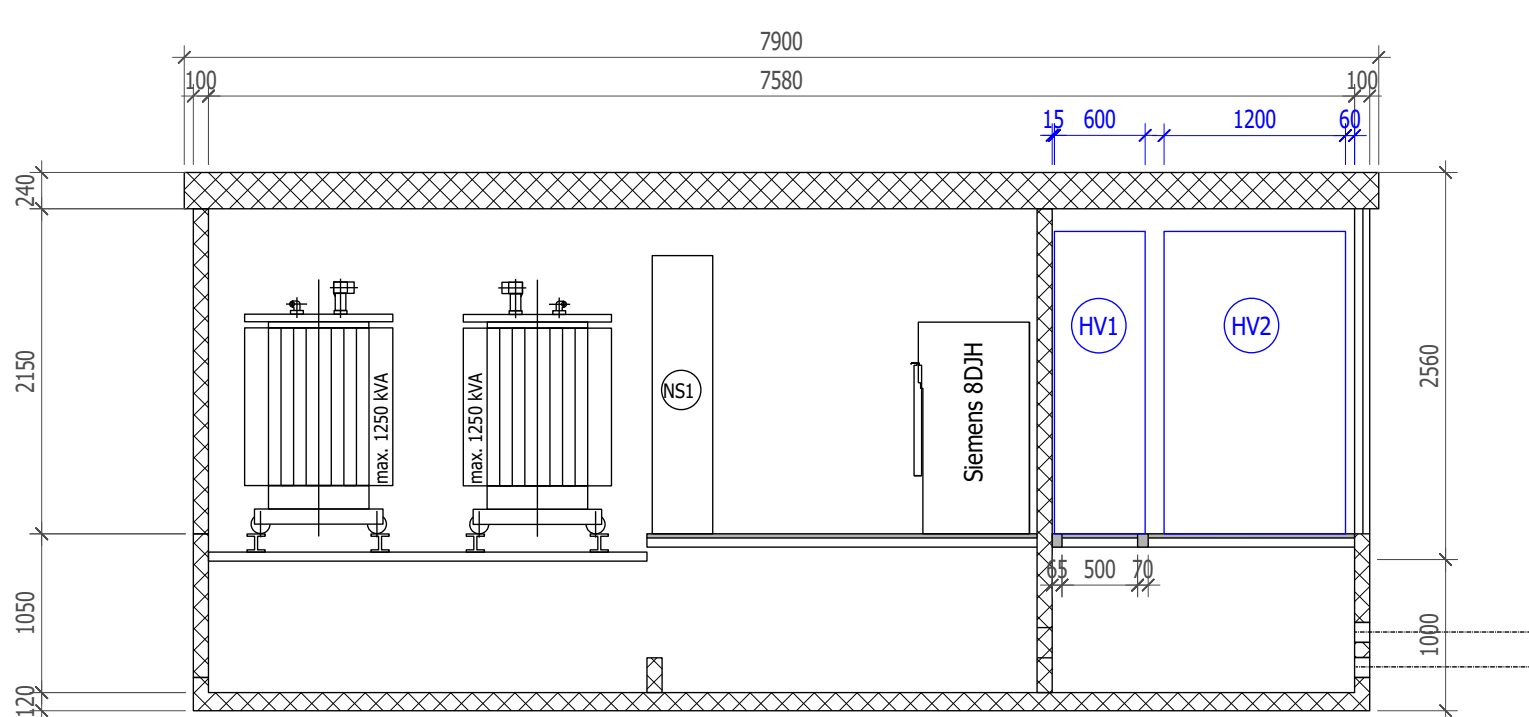
Schnitt D-D
