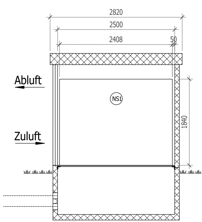
Schnitt B-B
