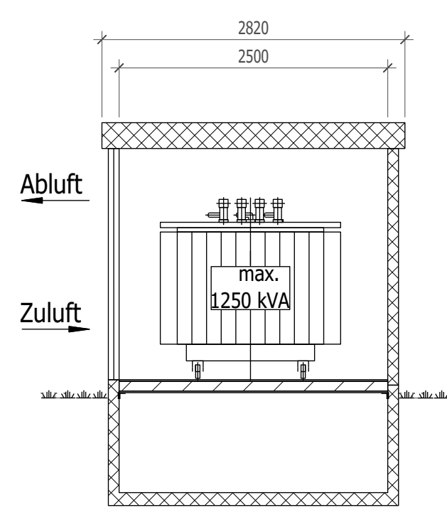
Schnitt A-A
