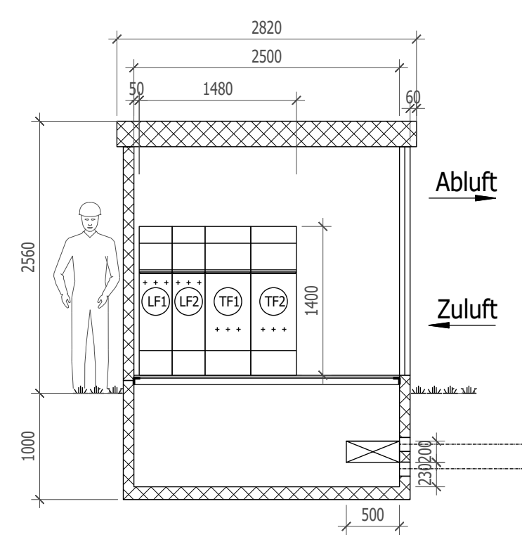
Schnitt C-C
